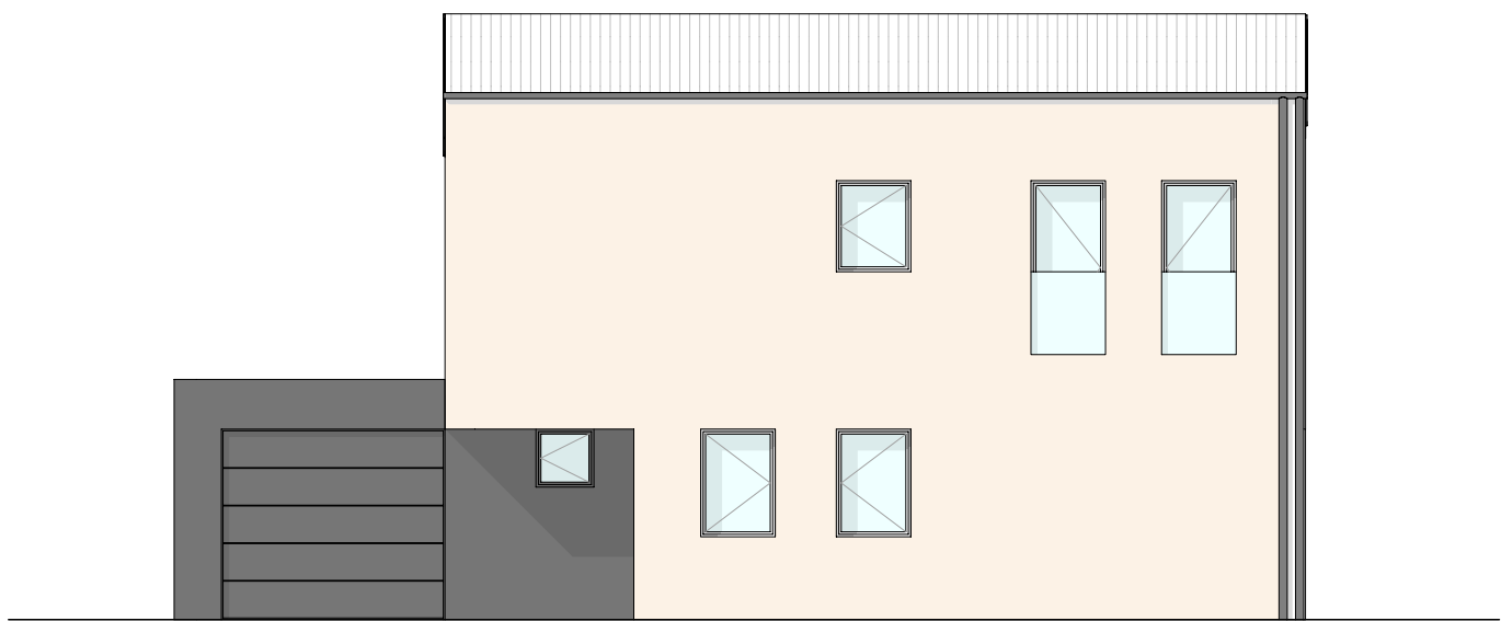
PROSPETTO NORD
