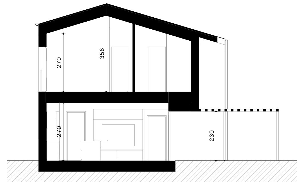
SEZIONE A-A'
