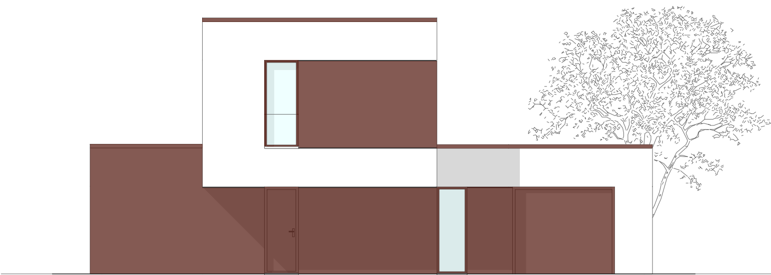
PROSPETTO EST
