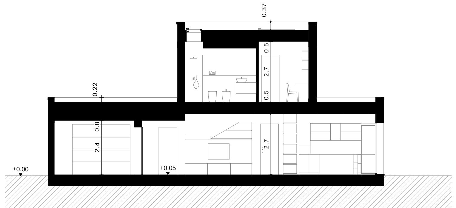
Sezione A-A'
